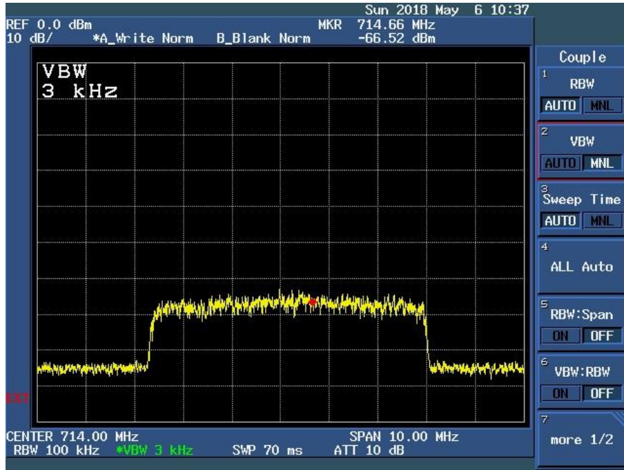
写真 1 JA0RUZ -66dBm SN 19dB 程度 (LO 551MHz)
