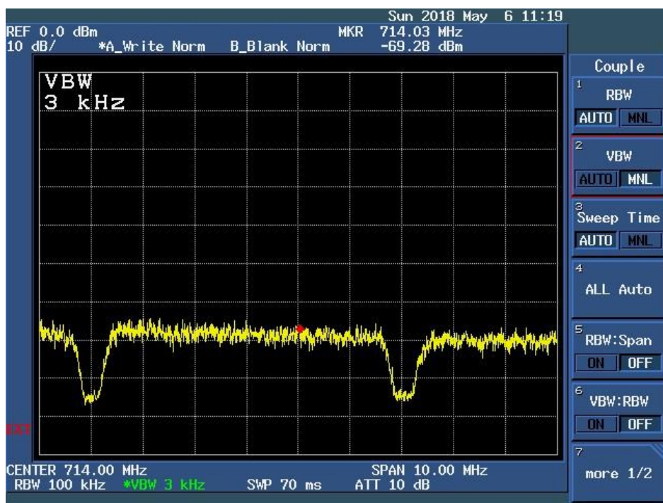
写真3 宅内のTV用 地デジの信号を見ると -69dBm SNは16dB程度
