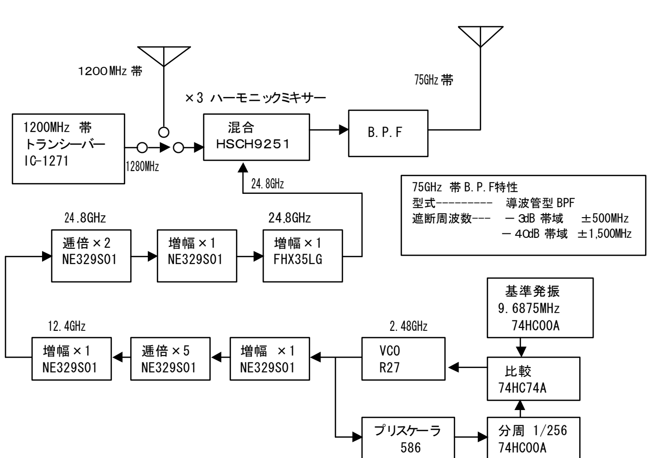
(別図-6) 75GHz帯ブロック図
