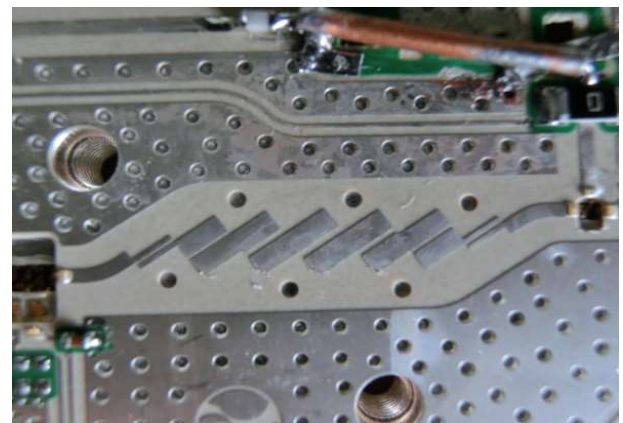
RF BPF カット
