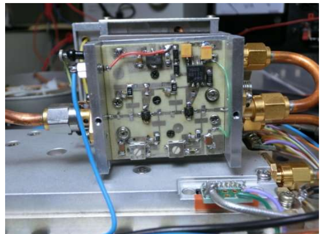
LNA
