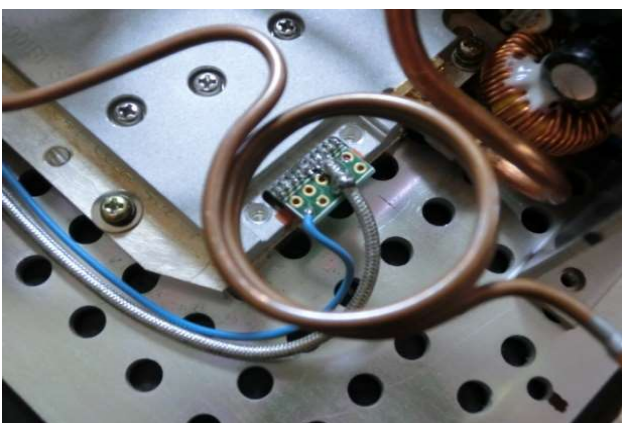
RX OUT コネクタ
