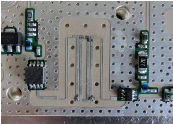
ダブル BPF スタブ付け
