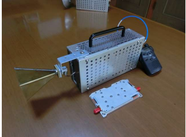
Ver-3 & WAVELAB 本体
