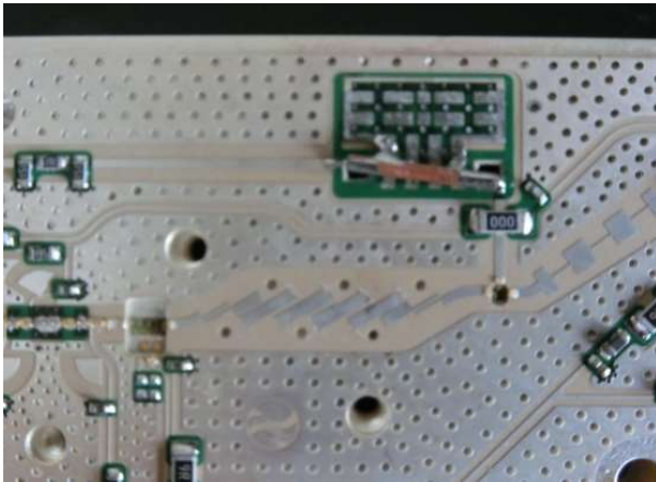
TX IF BPF 同軸ケーブル配線
