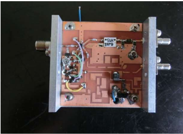
電源制御部
