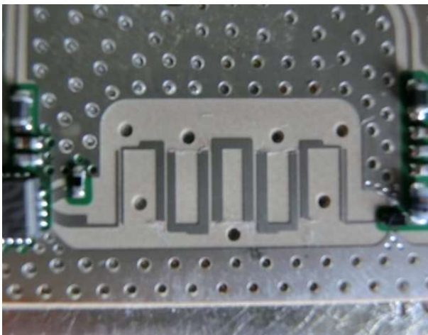
トリプラー-BPF カット
