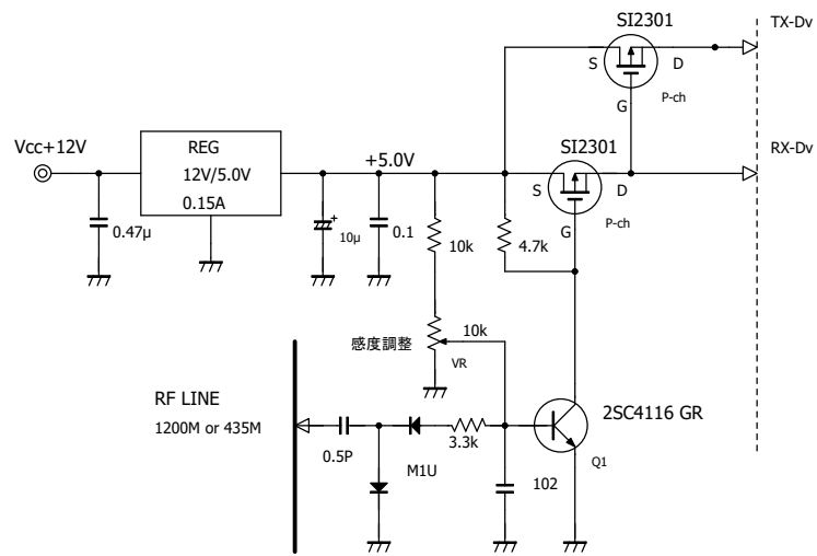
キャリアコン回路 Ver-1
