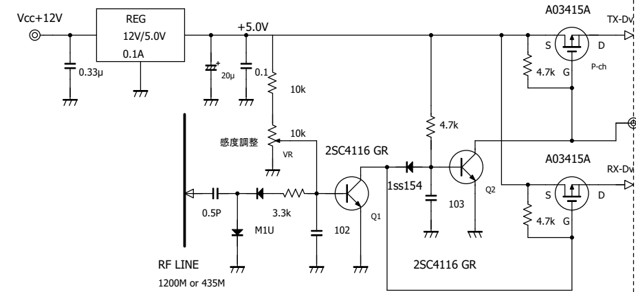
キャリアコン回路 Ver-2
