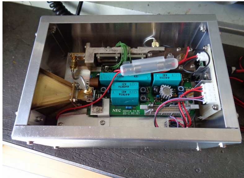
写真3. ケース組み込み
