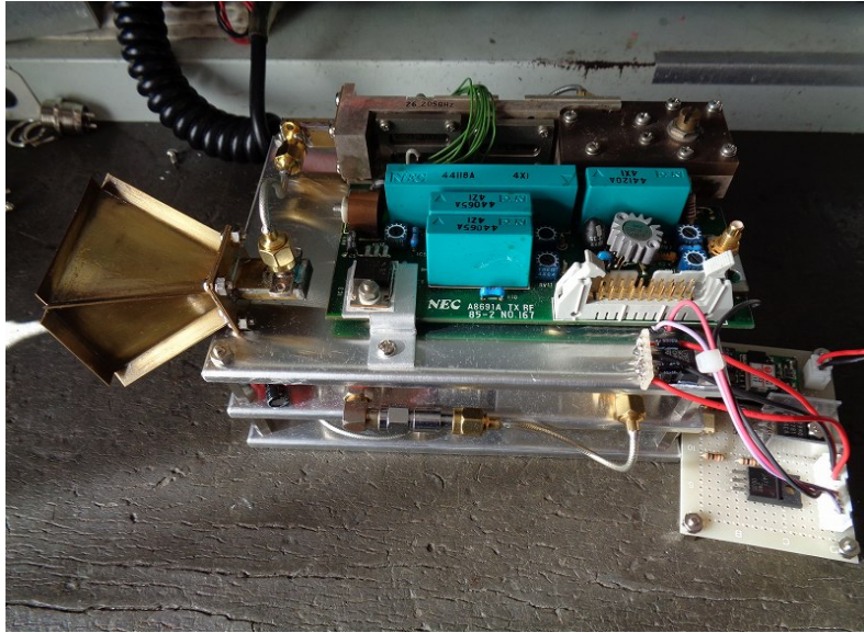
写真1. ビーコン内部
