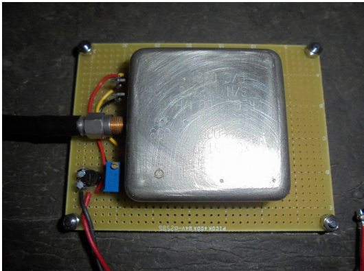
100MHz OCXO
