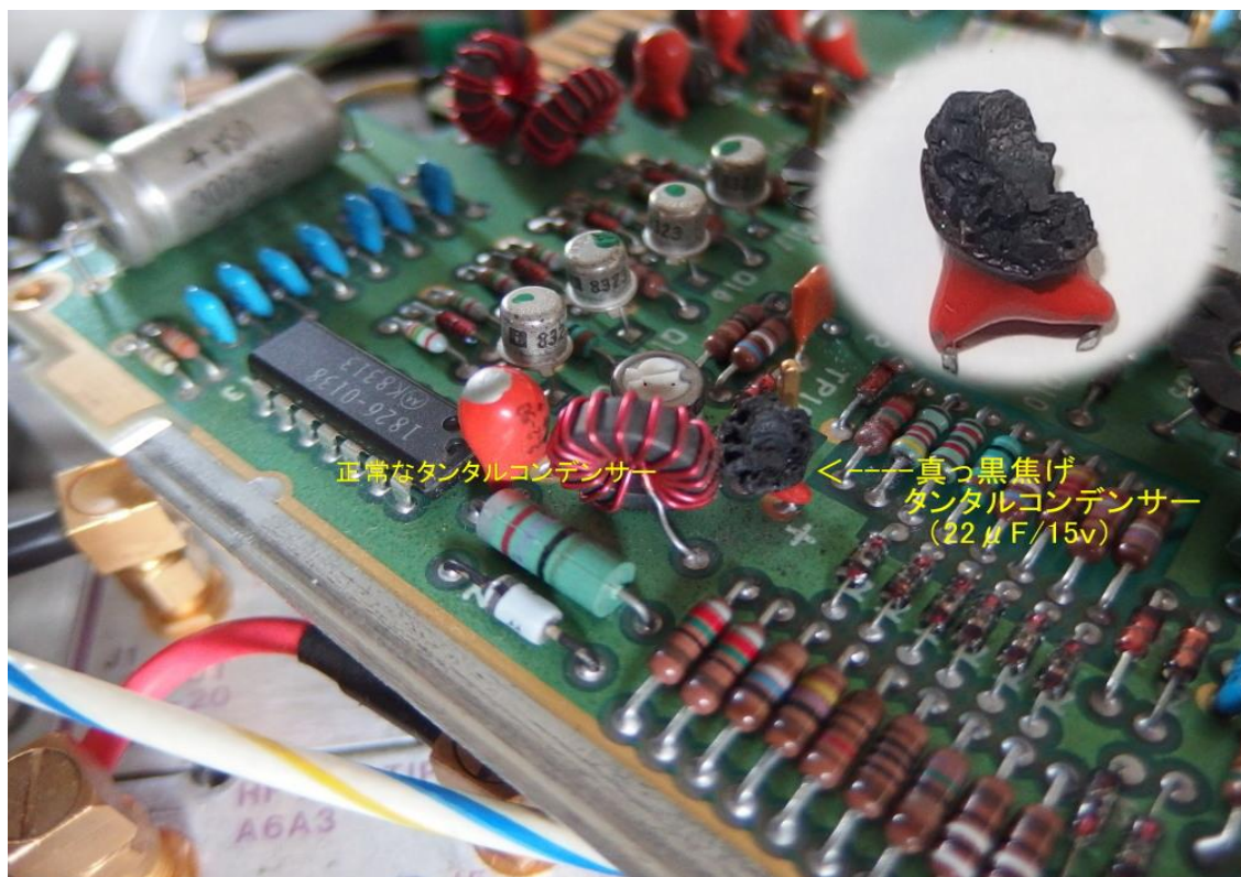
故障箇所 A6A5 C48 タンタルコンデンサー—22 μ /15v
