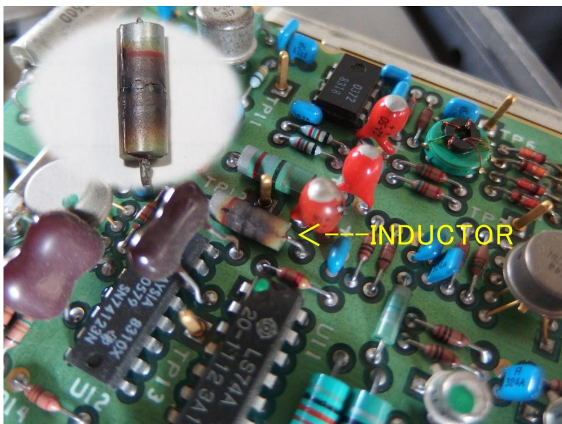
故障箇所 A6A5 L12 インダクター—27 μH
